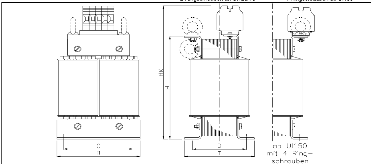
2 Ringschrauben an UI120/75
